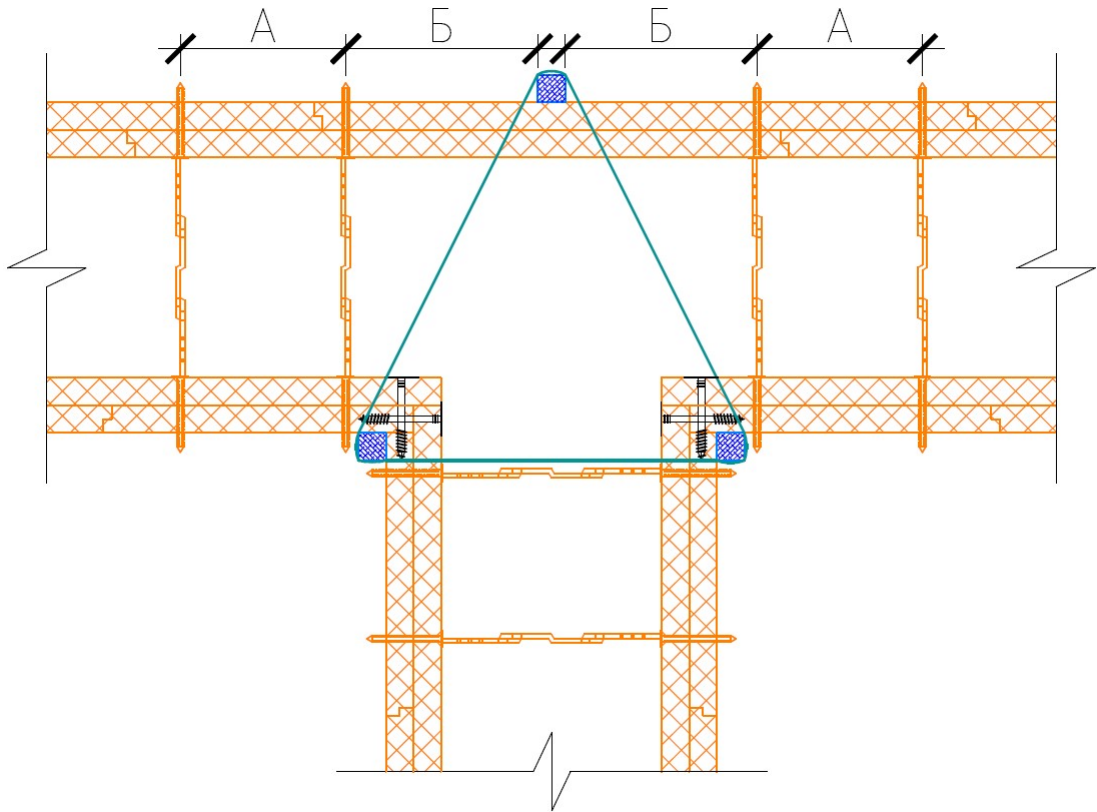
Рис. 5 Схема укрепления Т-образных углов опалубки
